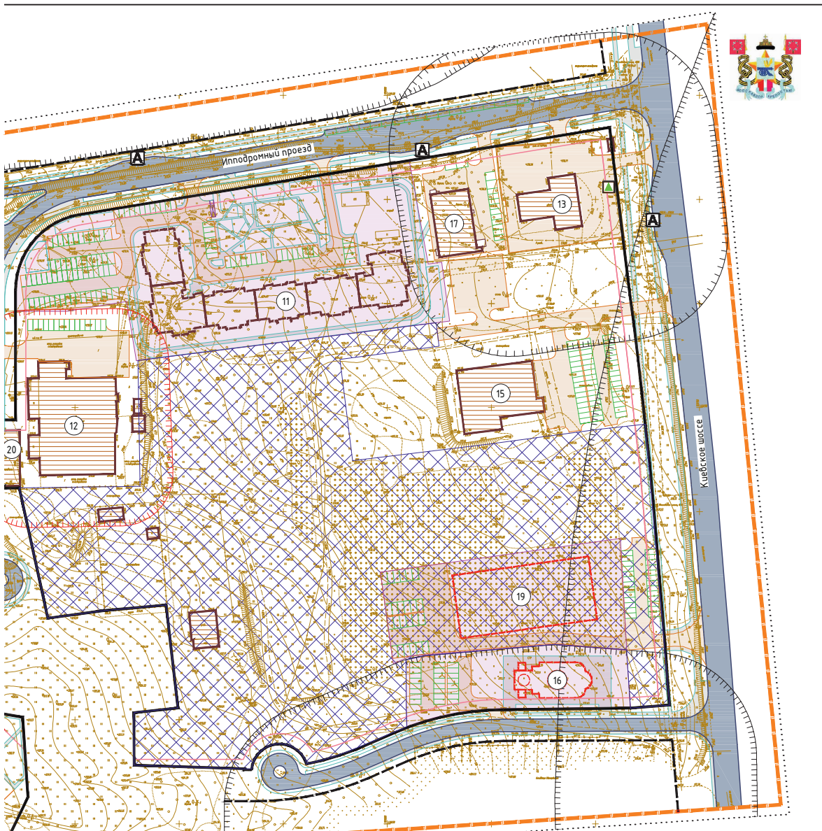
Экспликация объектов капитального строительства
